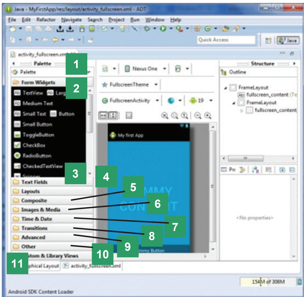
Εικόνα 7.2. Περιβάλλον ανάπτυξης εφαρμογών για φορητές συσκευές με Android
