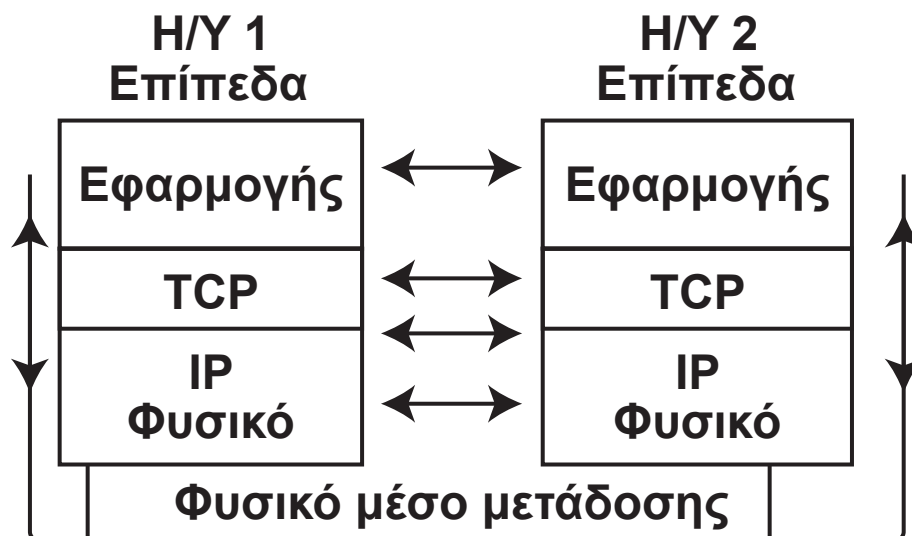
Εικόνα 9.2. Η λειτουργία του πρωτοκόλλου TCP/IP
