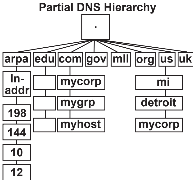
Εικόνα 9.3. Ιεραρχία DNS
